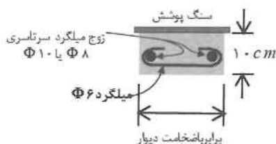
برابری ضخامت دیوار
