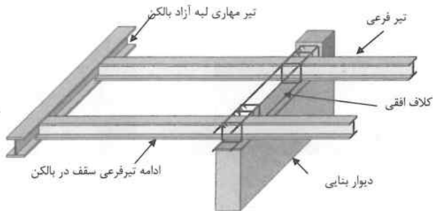
الف- تیر فرعی سقف عمود بر دیوار
