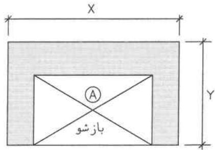
پ-۱ نامنظمی دیافراگم (درمساحت)
